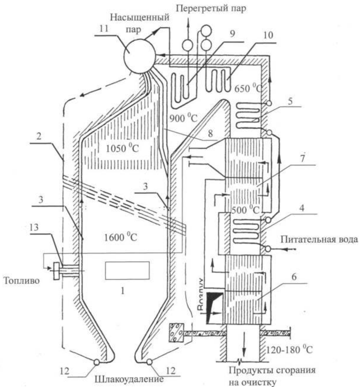
Рисунок 2.4 – Принципиальная схема парового котла
